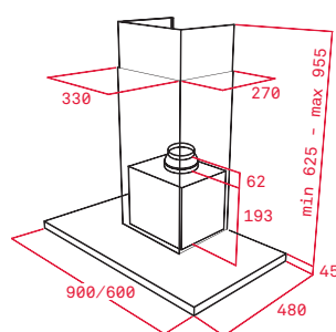
PERFECTA4 DLH 985 T | DH 680/980 T
