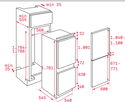
CI3 342 | CI3 350 NF
