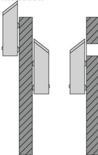
Első és/vagy felső és hátsó bedobónyílással is rendelkező modellek
