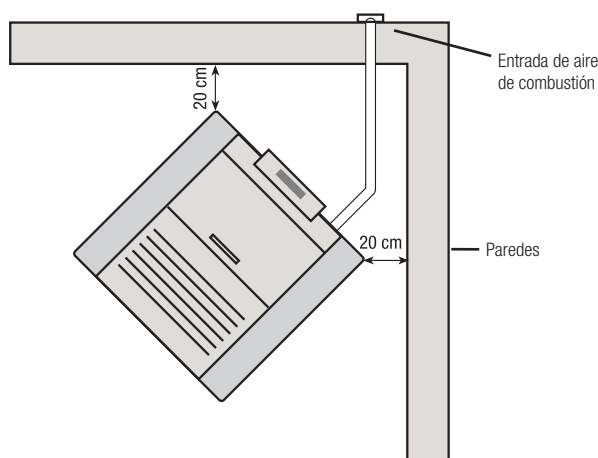
Imagen 6: Distancia desde las paredes
