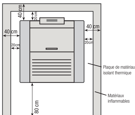
Fig. 5 distances minimum des objets
