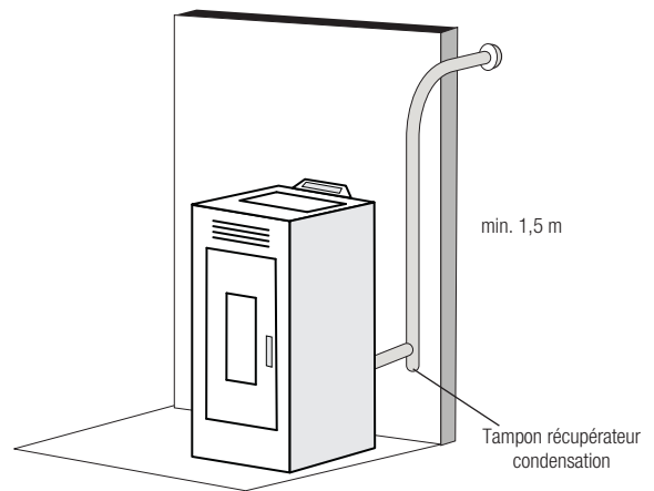
Fig.3: L'installation du tuyau d'évacuation de la fumée doit être aux termes de loi.
