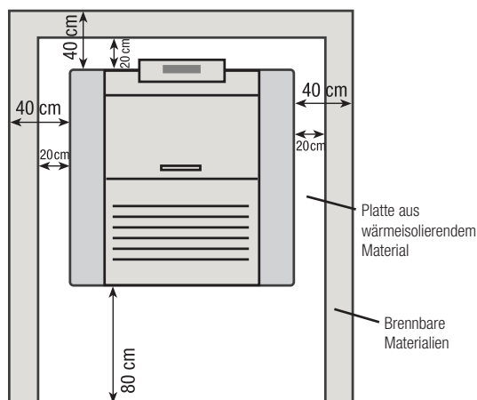
Bild 5: mindeste Sicherheitsabstände
