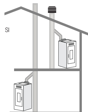
Fig.1: metodologie d'installazione della canna fumaria
