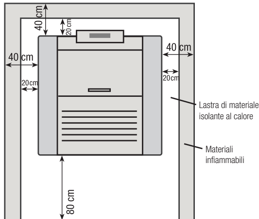
Fig. 5 distanze minime dagli oggetti
