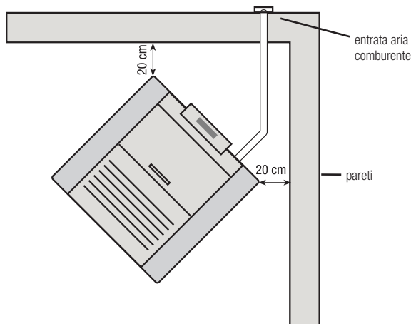
Fig. 6 distanze minime dalle pareti
