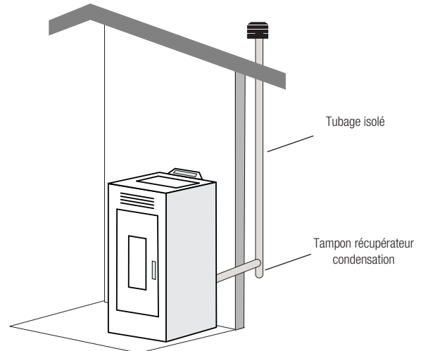
Fig.4: installation conduit de fumées externe
