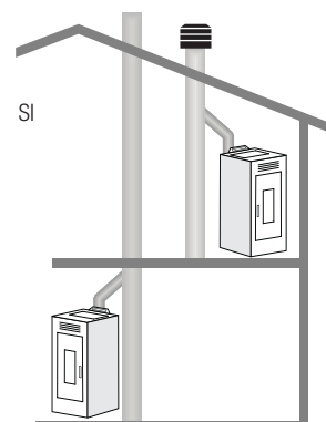
Imagen 1: Métodos para instalar la salida de humos
