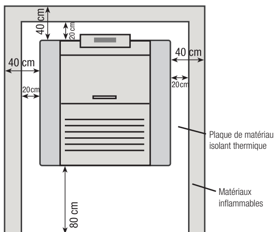
Imagen 5: Distancia mínima de los objetos.
