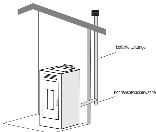
Bild 4: Installation der äußeren Schornsteins
