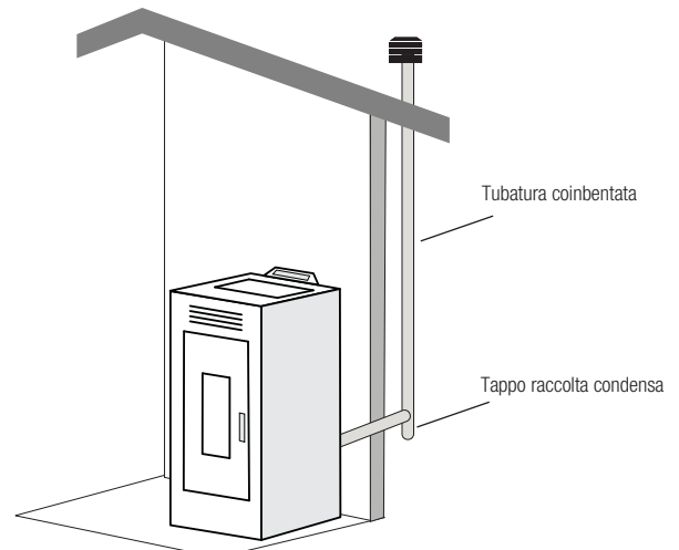
Fig. 4: installazione canna fumaria esterna
