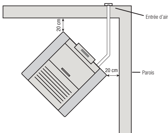
Fig. 6 distances des murs
