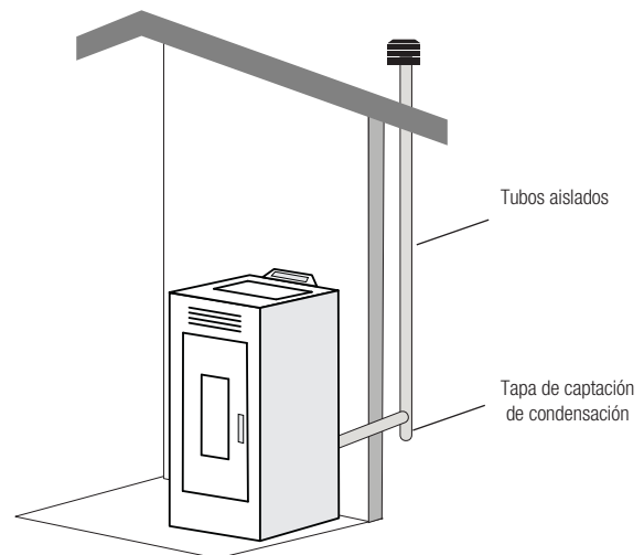
Imagen 4: instalación de combustión externa
