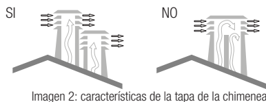
Imagen 2: características de la tapa de la chimenea
