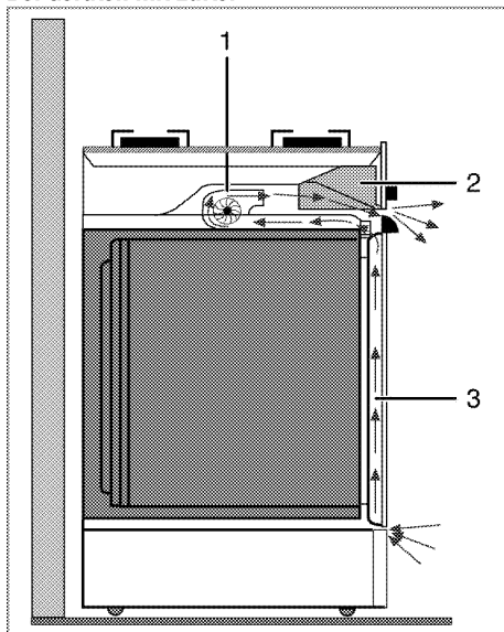
1 Lüfter
