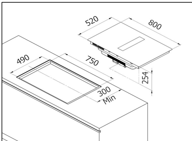
Installazione in appoggio / Non-Flush installation
