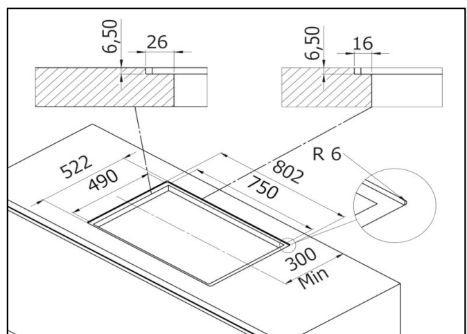
Installazione a filo / Flush installation
