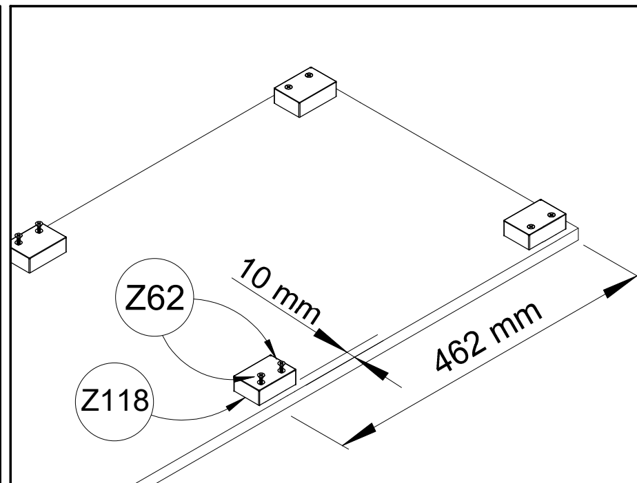
Šablona pro montáž kluzáků Schablone für die Gleitermontage
