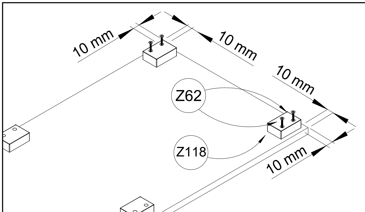
Šablona pro montáž kluzáků Schablone für die Gleitermontage
